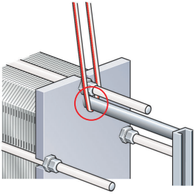
Figure 6 : Levage des modèles M3, M6, M10, T2, T5, TL3 et de l'ancienne version du modèle T8, TL6
