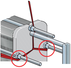
Figure 7 : Levage du modèle TS6.
