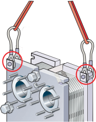
Figure 8 : Levage des modèles T10, T6, T8, TL6
